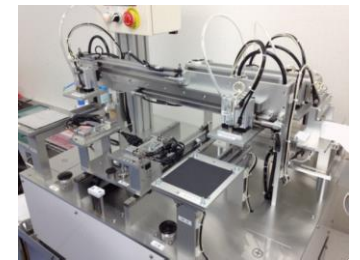
電極積層機
