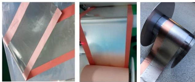
負極集電箔(Li/LiCu/LiCuLi)
